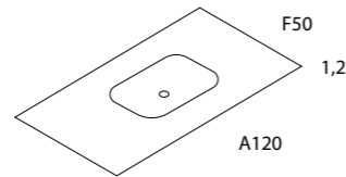
ENCIMERA Fabricada en Solid Surface Acabado Blanco Lavabo TAP60 Posición Seno Central
